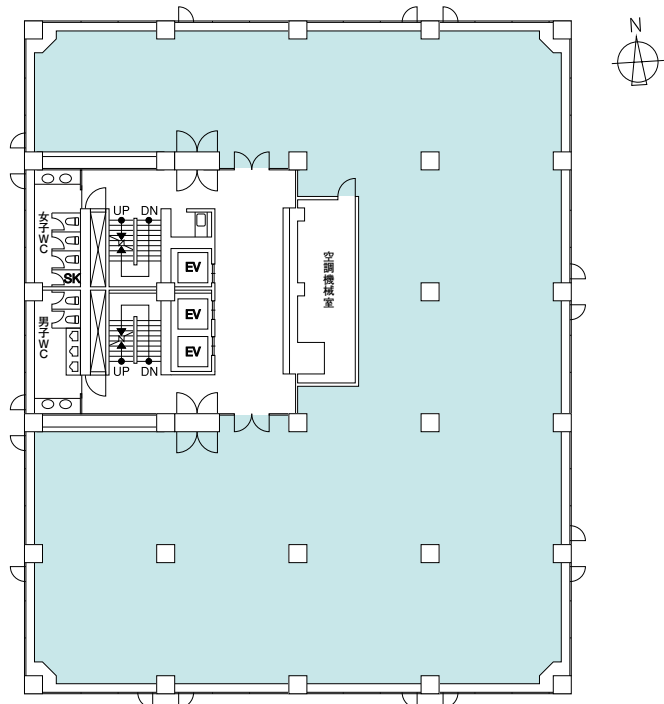
フロア(基準階)
